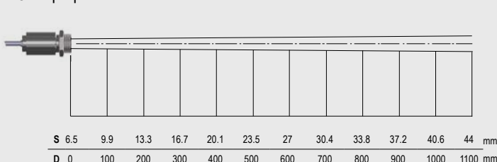
25:1 optique
