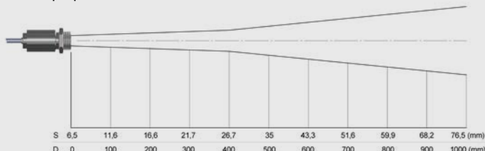
15:1 optique
