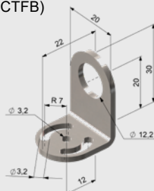
Equerre de montage, fixe (ACCTFB)
